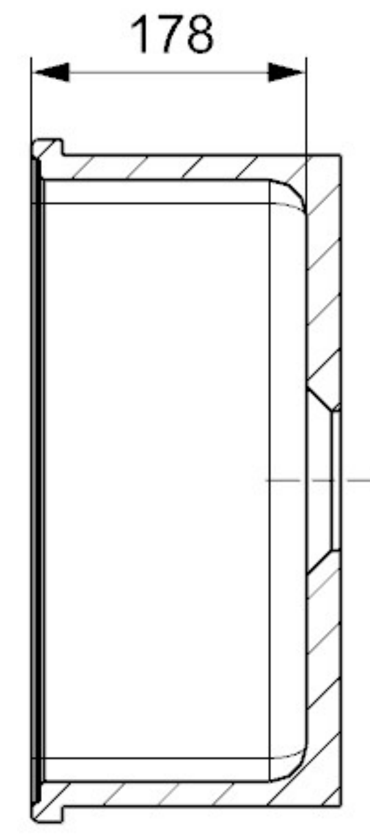
SECTION A-A
